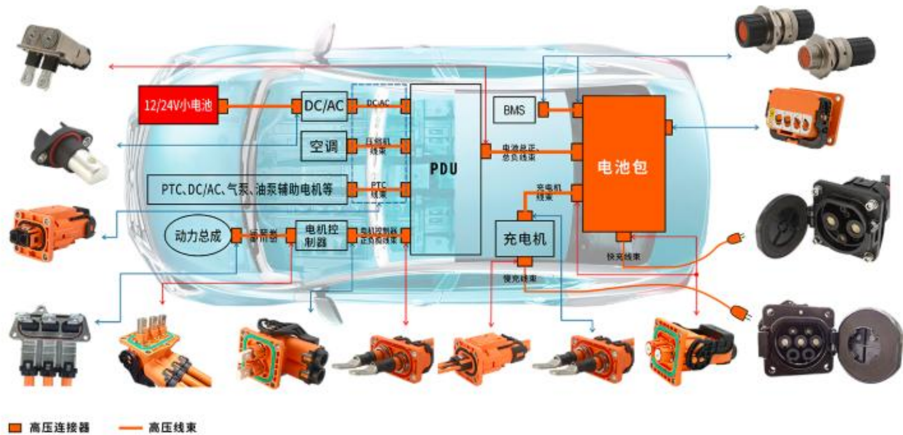
乘用车高压连接器解决方案
